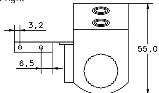
Seitenansicht von rechts side view right
