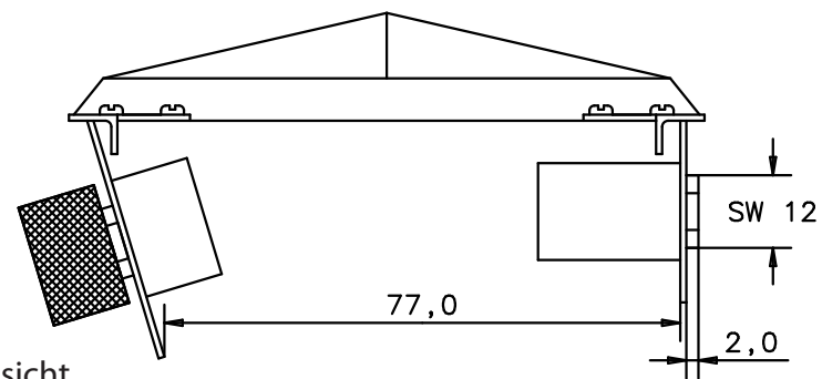
Unteransicht bottom view
