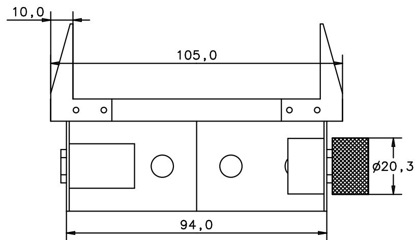
Seitenansicht von rechts side view right
