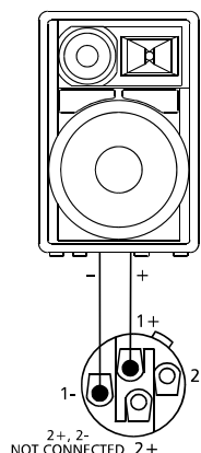
Abbildung 2-19: Anschlussbeispiel einer passiven Lautsprecherbox
