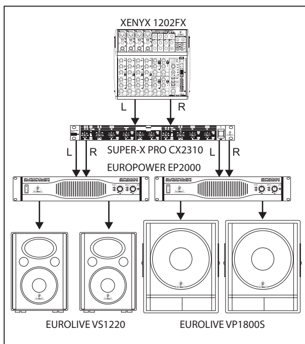
Abb. 5.3 2-Weg Stereobetrieb mit Subwoofern
