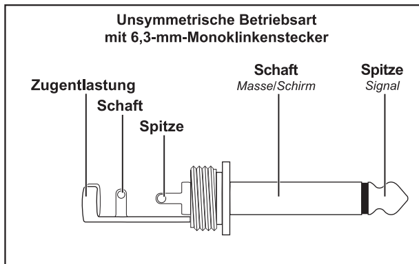
Abb. 2.3 1/4" TS Boxenanschluss
