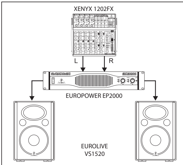
Abb. 5.1 Breitbandiger Stereobetrieb
