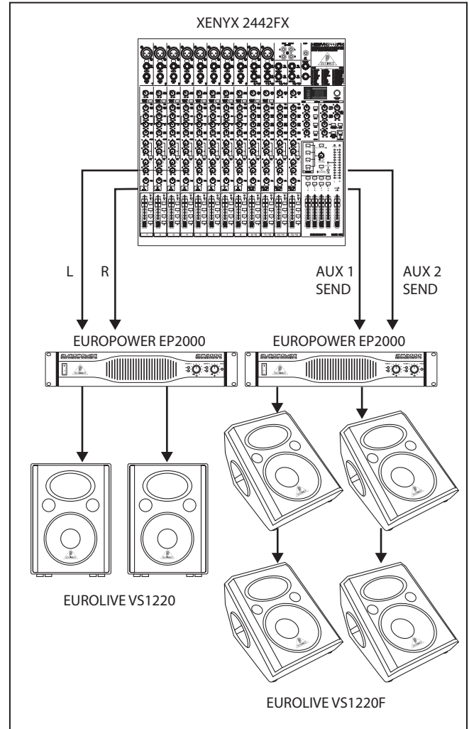
Abb. 5.2 2-Breitband-Stereobetrieb mit Bodenmonitoren
