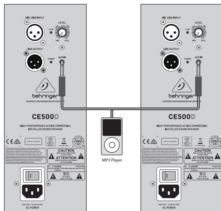
Connecting a stereo signal source Conexión de una fuente de señal stereo Connexion d'une source stéréo Stereosignalquelle anschließen Conectando una fonte de sinal estéreo
