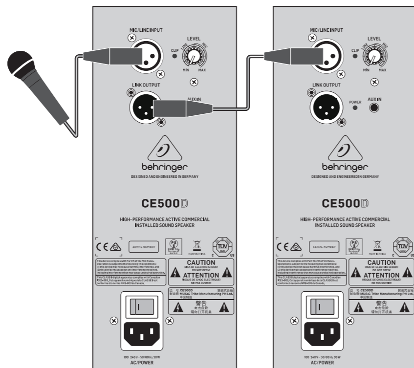
Connecting a microphone Conexión de un micrófono Connexion d'un micro Mikrofon anschließen Connecting a microphone
