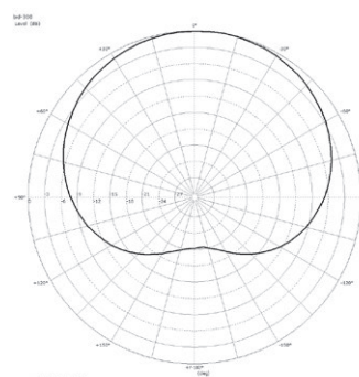
Polardiagramm @ 1 kHz
