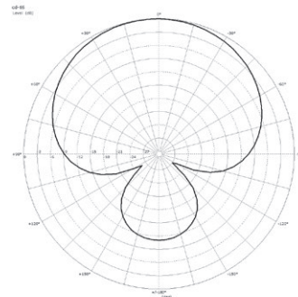
Polardiagramm @ 1 kHz
