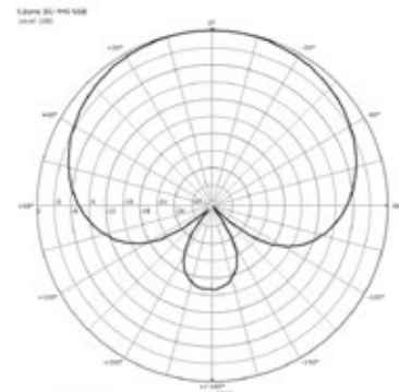
Polardiagramm @ 1 kHz
