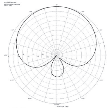
Polardiagramm @ 1 kHz
