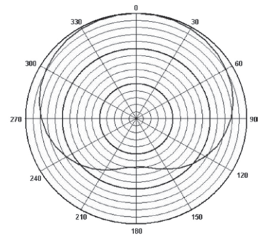
Polardiagramm @ 1 kHz
