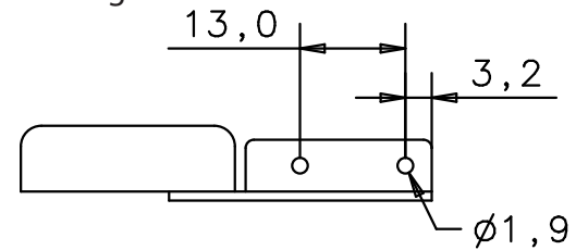
Seitenansicht von rechts side view right
