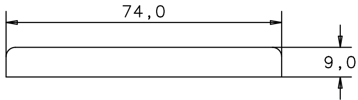
Vorderansicht front view
