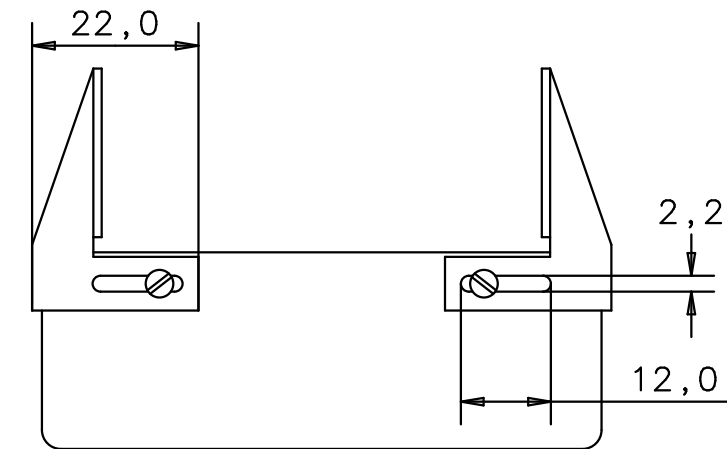
Seitenansicht von rechts side view right
