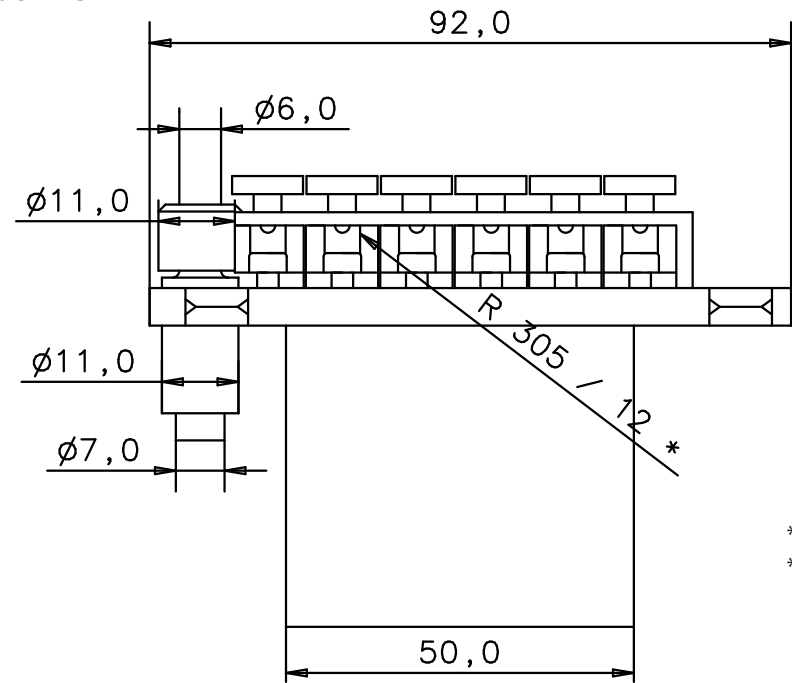
Rückansicht back view
