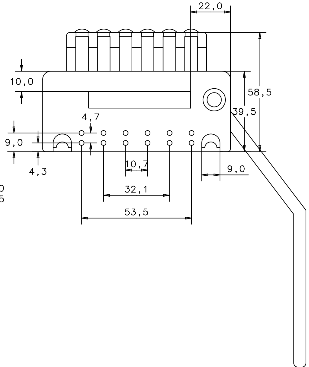
Untersicht bottom view
