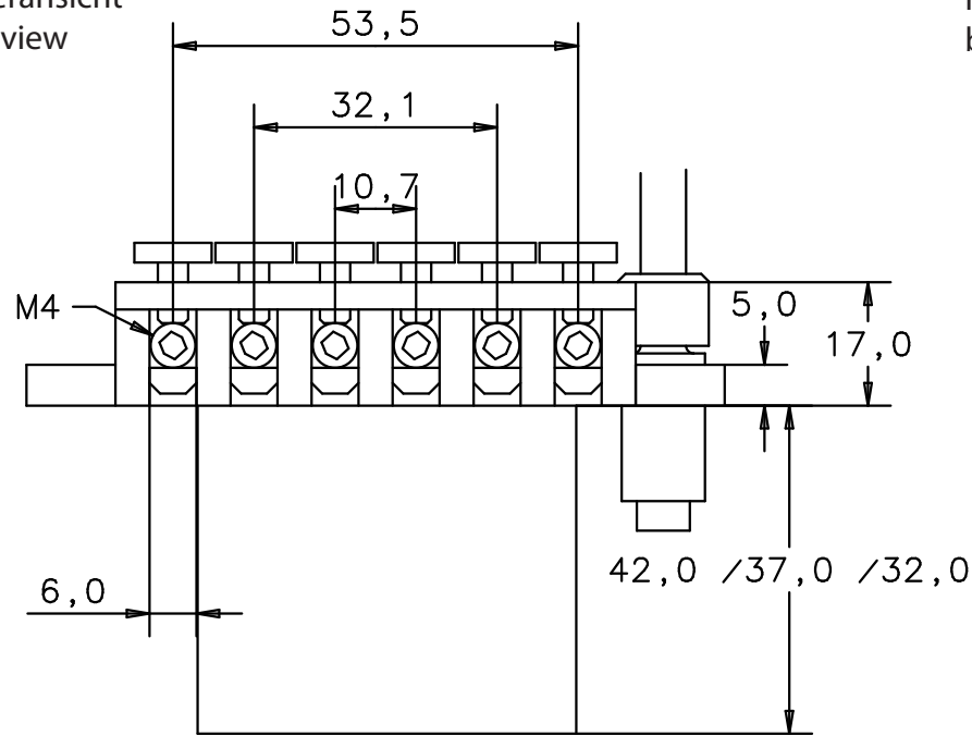
Seitenansicht von links side view left
