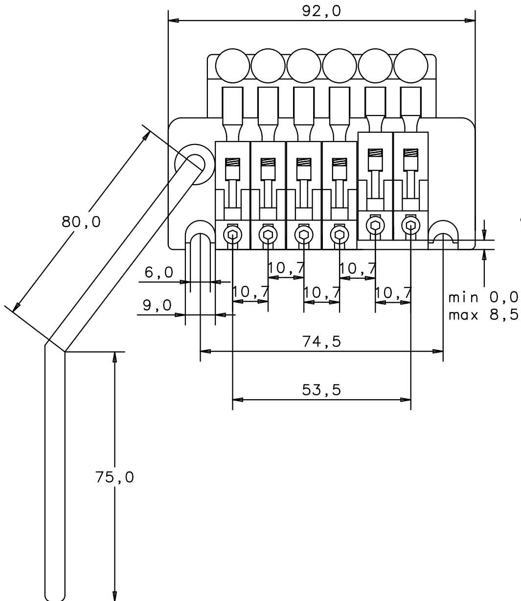
Draufsicht top view
