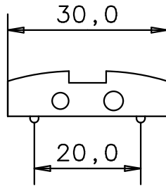
Vorderansicht front view
