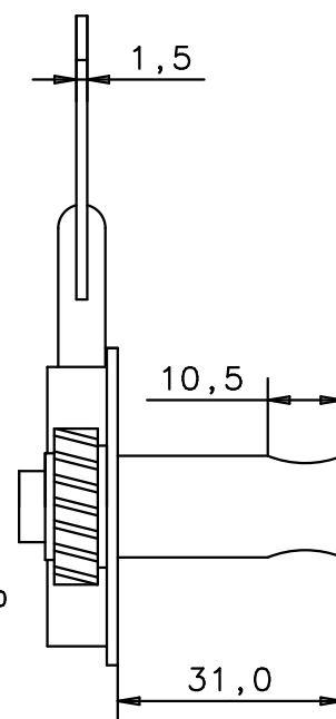
Seitenansicht von links side view left
