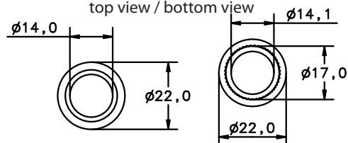
Draufsicht / Untersicht top view / bottom view
