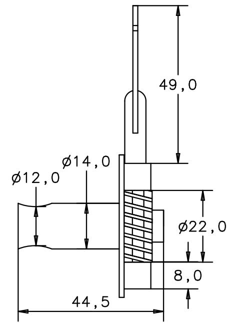
Seitenansicht von rechts side view rechts
