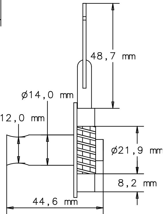
Seitenansicht - links side view - left
