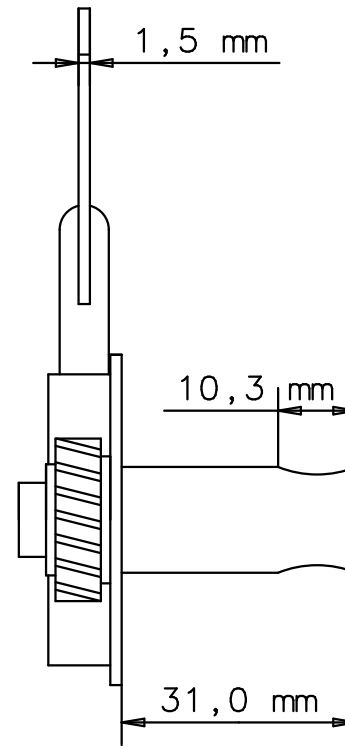
Seitenansicht - rechts side view - right
