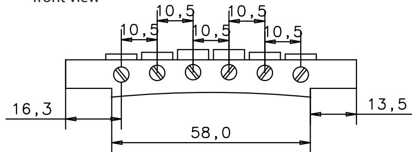
Vorderansicht front view
