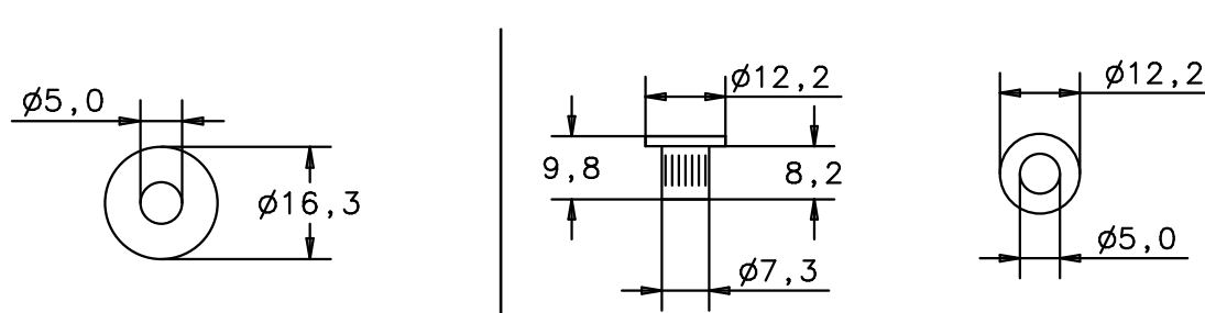
Höhenverstellungsschraube level adjustable screw
