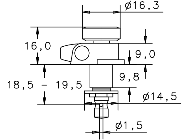
Untersicht bottom view
