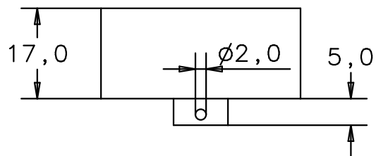
Seitenansicht von links side view left
