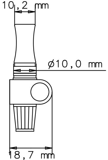
Seitenansicht - rechts side view - right
