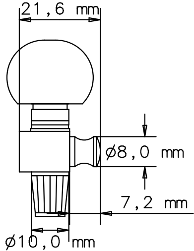
Rückansicht back view
