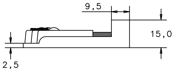
Seitenansichten side views
