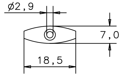
Untersicht bottom view
