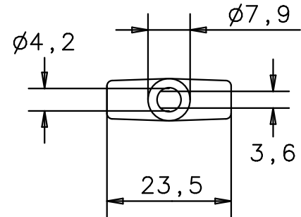
Untersicht bottom view
