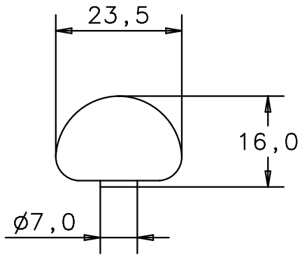
Vorderansicht / Rückansicht front view / back view
