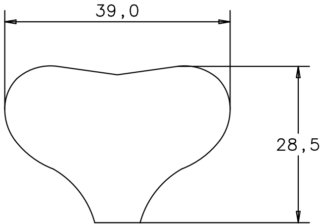
Vorderansicht / Rückansicht front view / back view
