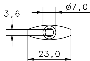
Untersicht bottom view
