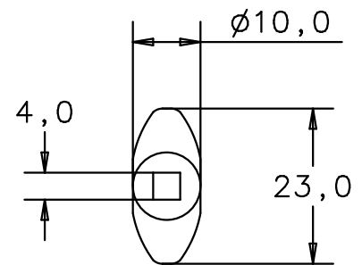
Untersicht bottom view
