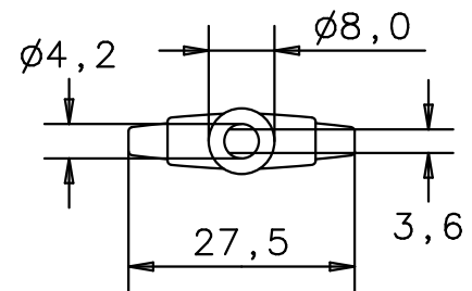
Draufsicht top view
