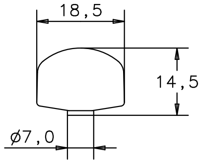
Vorderansicht / Rückansicht front view / back view
