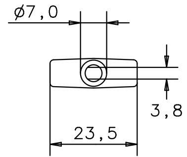
Untersicht bottom view
