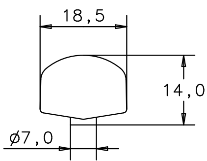
Vorderansicht / Rückansicht front view / back view
