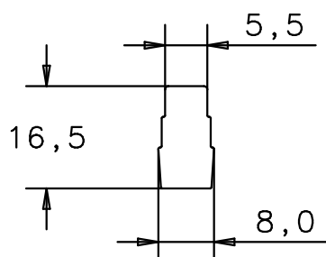
Seitenansicht side view
