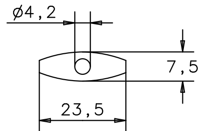
Untersicht bottom view
