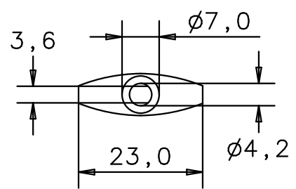
Untersicht bottom view
