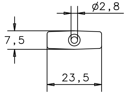
Draufsicht top view
