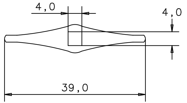
Draufsicht top view
