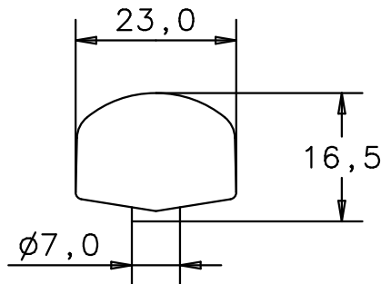
Vorderansicht / Rückansicht front view / back view
