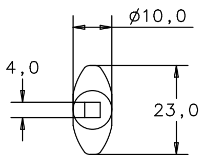
Untersicht bottom view
