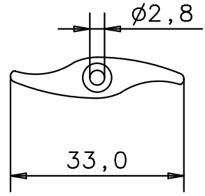
Untersicht bottom view
