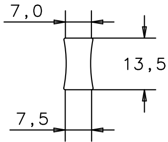
Seitenansicht side view
