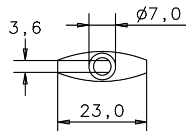
Untersicht bottom view
