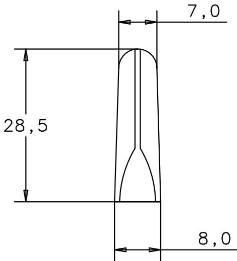
Seitenansicht side view
