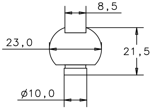
Vorderansicht / Rückansicht front view / back view
