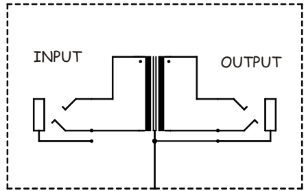
SCHALTSCHHEMA PLI01
