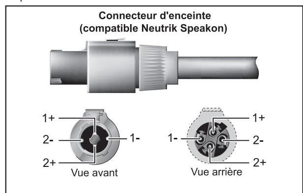
Fig. 1.3: Connecteur Speakon
