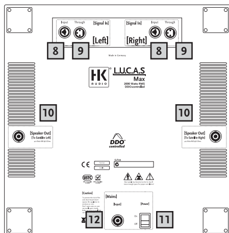
L.U.C.A.S MAX - Bedienfeld Rückseite
