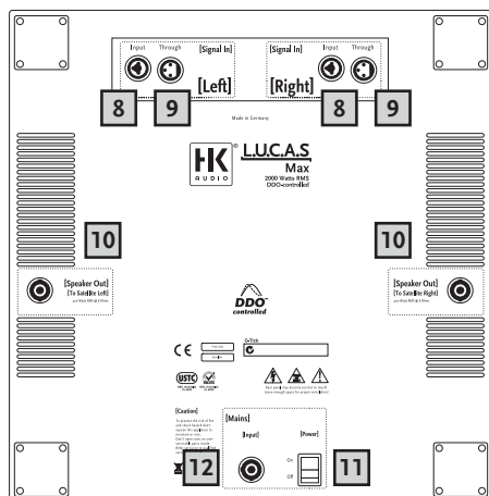
L.U.C.A.S MAX - Subwoofer
