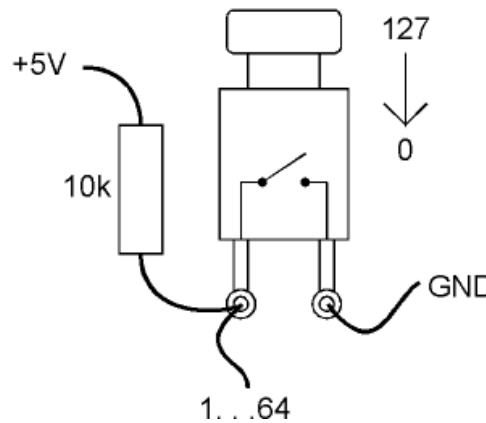
Anschluss eines Tasters oder Schalters ( Variante 2 )
