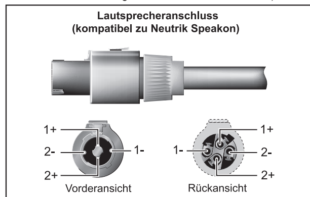
Abb. 1.3: Speakon-Stecker
