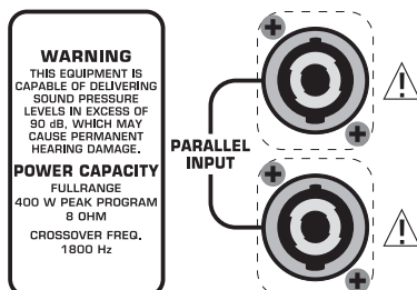
Abb. 1.1: Anschlussfeld der B1520 PRO (B2520 PRO/B1220 PRO ähnlich)
