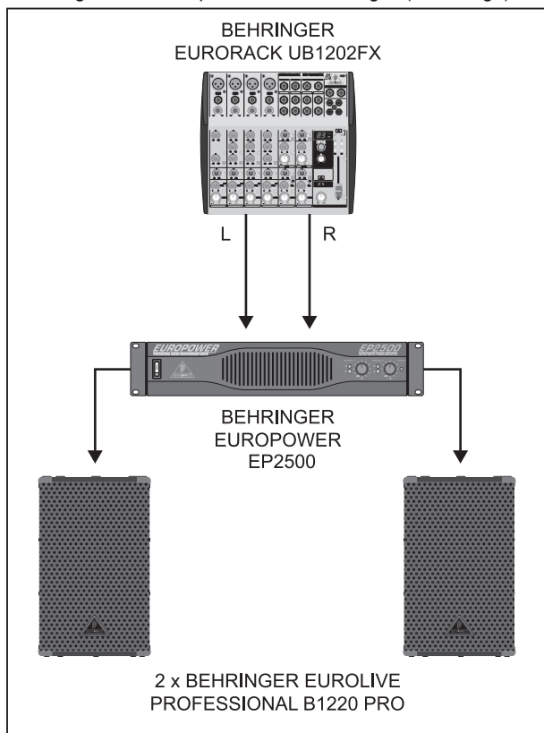
Abb. 6.1: Full Range-Stereobetrieb
