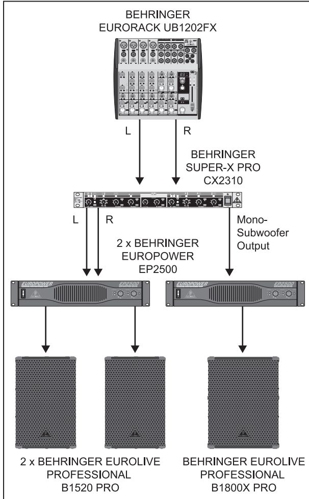
Abb. 6.2: Stereobetrieb mit Subwoofer
