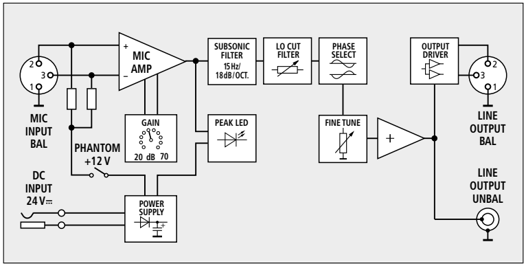
Blockschaltbild eines Kanals Block diagram of one channel
