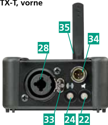
— TX-T, vorne
