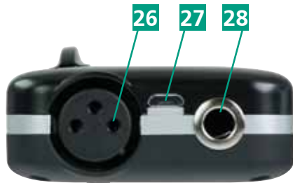
— TX unten
