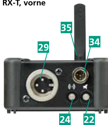
— RX-T, vorne
