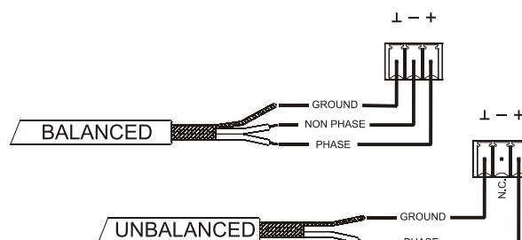
11. Connexions symétrique et asymétrique
