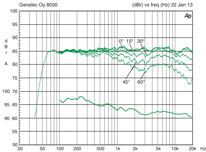
Abbildung 5. Die obere Kurvenschar zeigt die horizontale Abstrahlcharakteristik des 8030B gemessen in einem Meter Abstand. Die untere Kurve zeigt das Bündelungsmaß.
