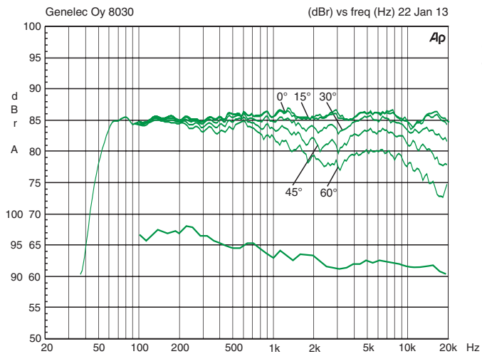
Illustration 5. Le groupe de courbes montre les caractéristiques de directivité horizontale de la 8030B mesurées à 1 m. La courbe inférieure montre la réponse en puissance de l'enceinte.
