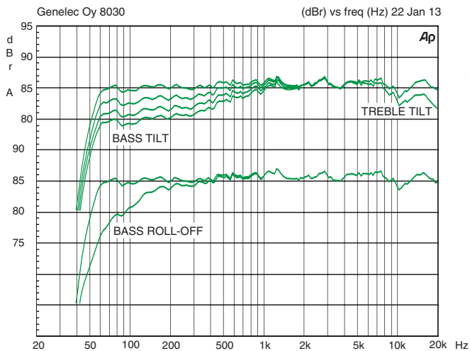
Illustration 4. Les courbes montrent l'effet des commandes "Bass Tilt", "Treble Tilt" et "Bass Roll-Off" sur la réponse en fréquence en champ libre de la 8030B.
