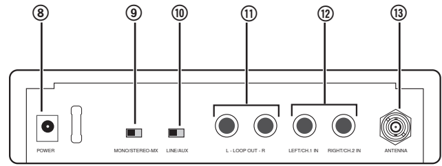
Rückseite des P3T
