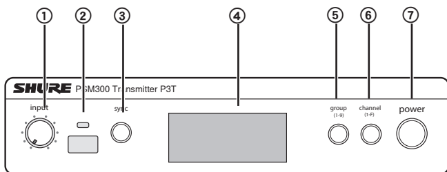
P3T-voorpaneel
