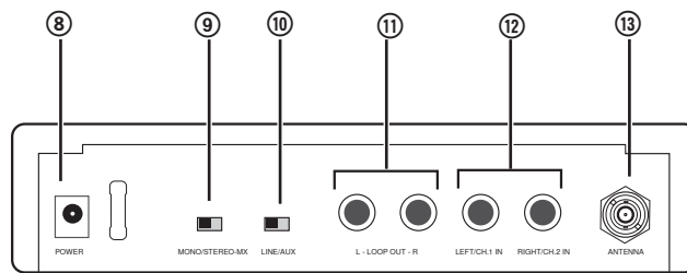
P3T-achterpaneel
