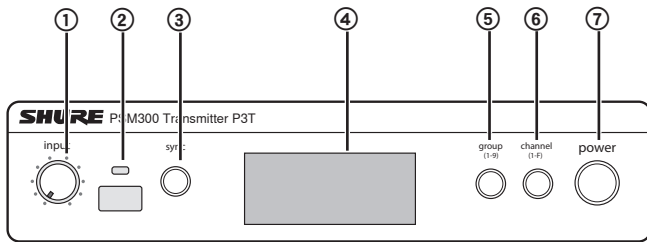
Vorderseite des P3T
