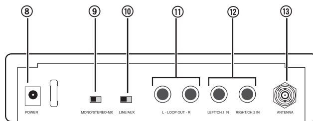
Pannello posteriore del P3T
