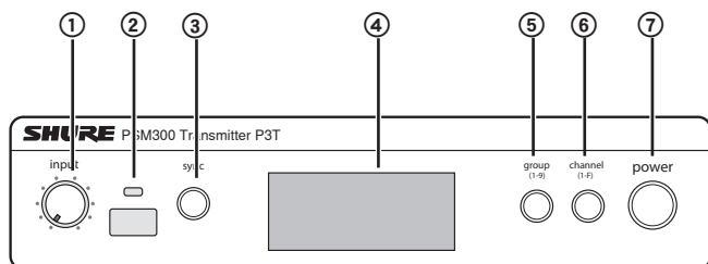
Передняя панель P3T
