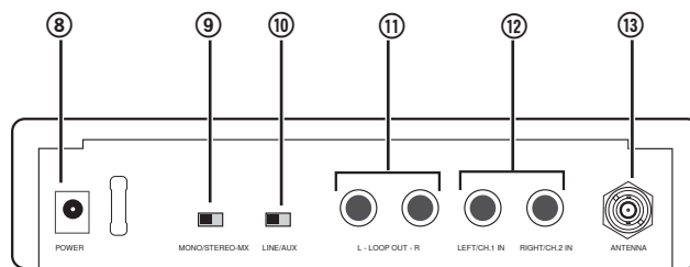
Задняя панель P3T
