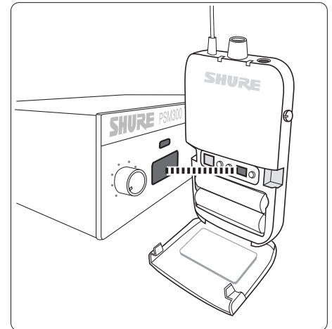
Alinhe as janelas de infravermelho para sincronizar o receptor e o transmissor
