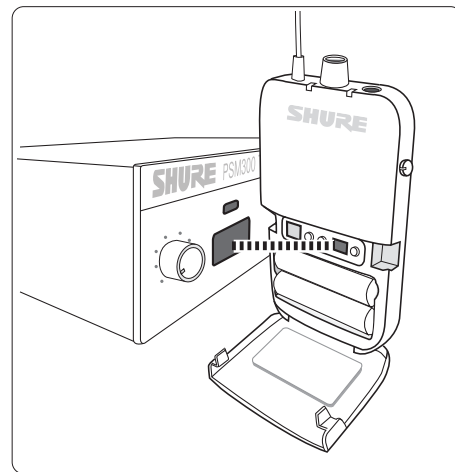
Для синхронизации приемника и передатчика направьте друг на друга их ИК окна.
