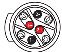
Cableado NL4 macho
