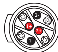
针式 NL4 线缆连接
