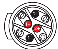
Câblage NL4 mâle
