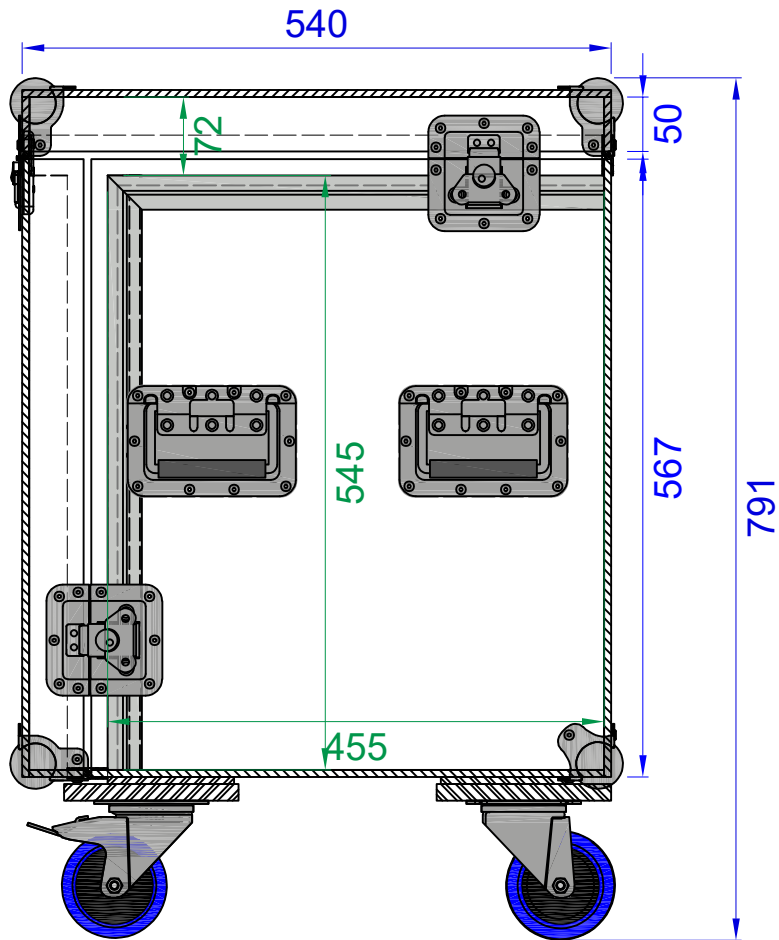
Seitenansicht / sideview
