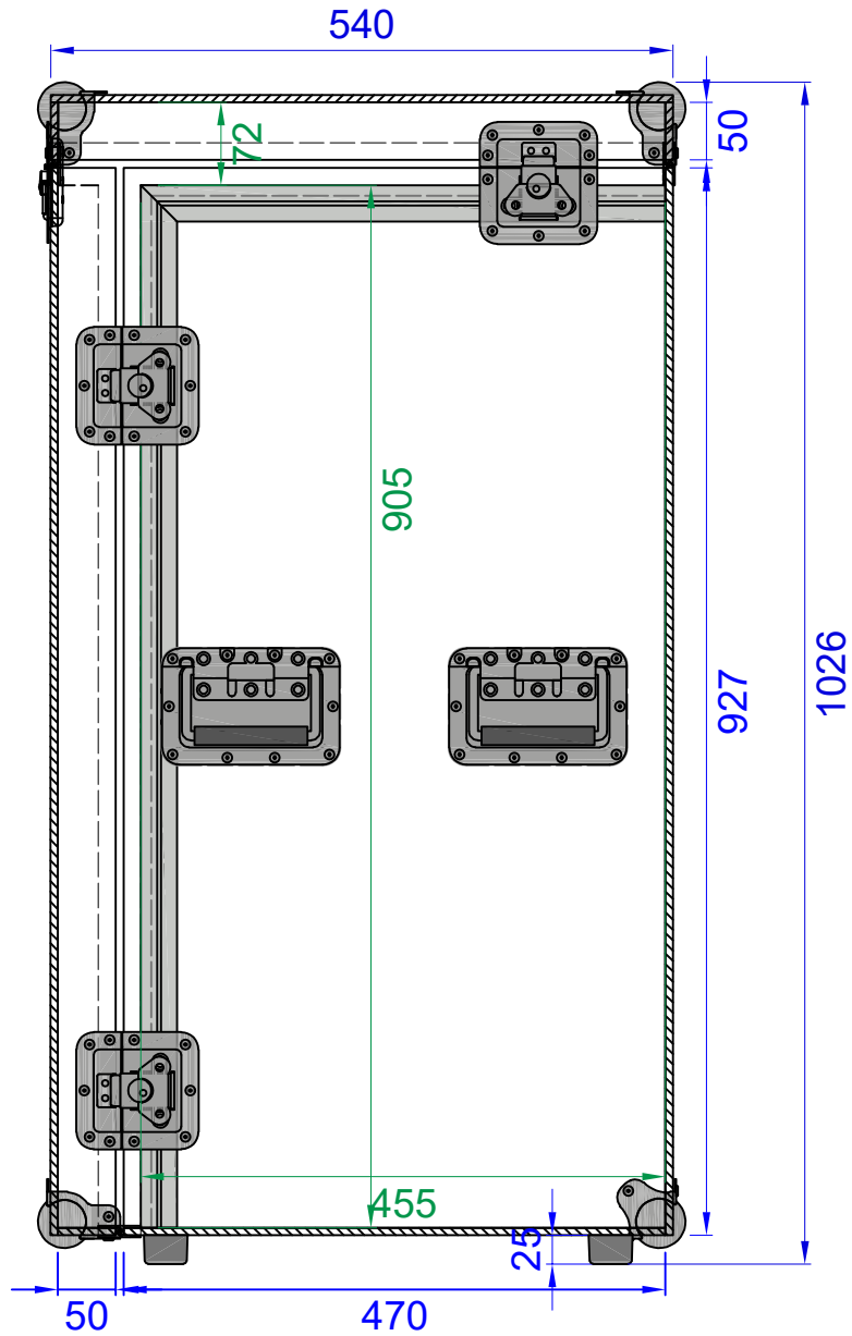
Seitenansicht / sideview
