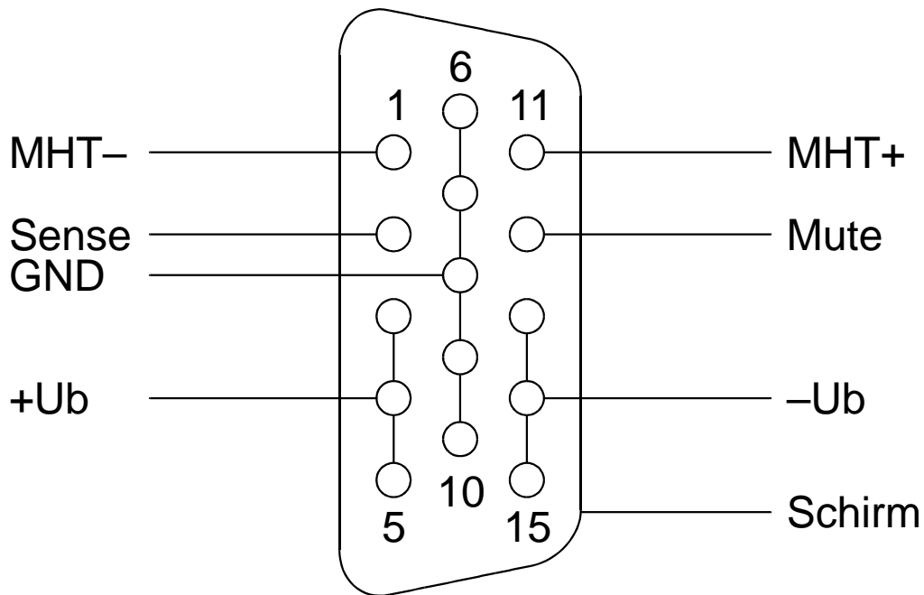
Pin-Belegungstabelle M3-220 Sub
