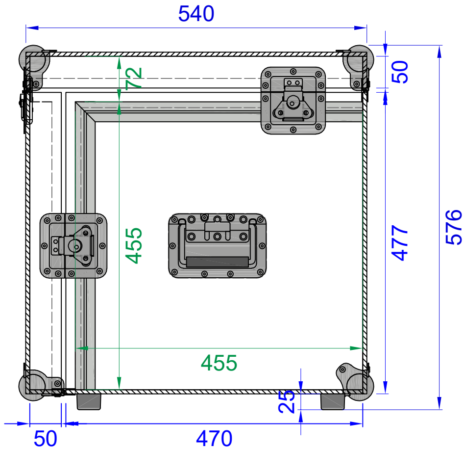
Seitenansicht / sideview
