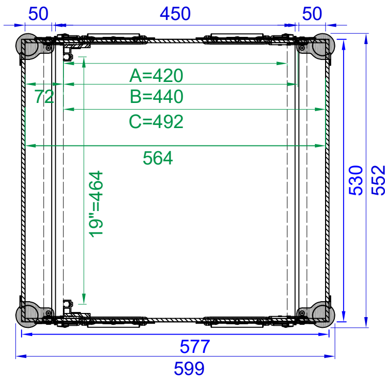
Draufsicht / topview
