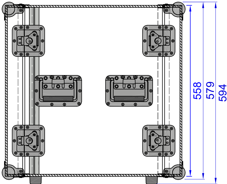
Seitenansicht / sideview
