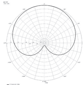
Polardiagramm @ 1 kHz
