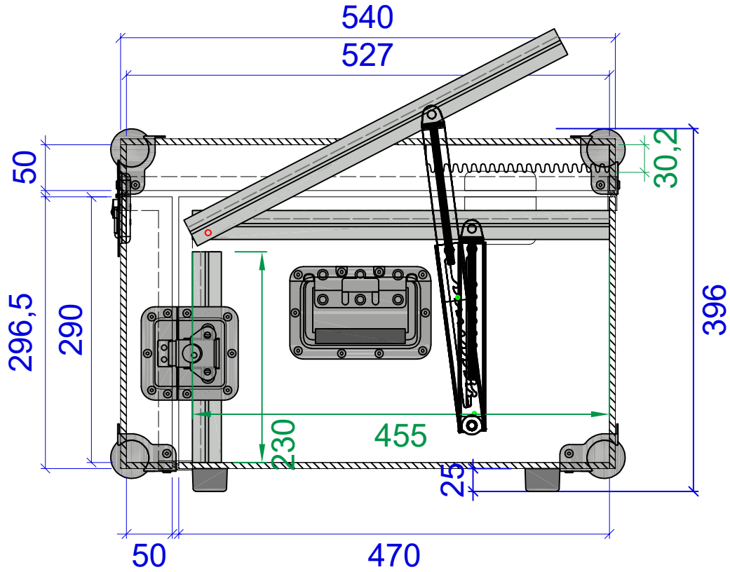
Seitenansicht / sideview
