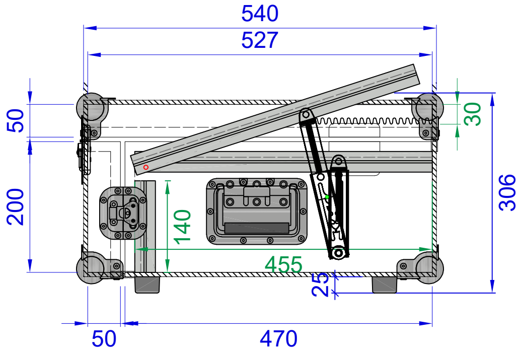
Seitenansicht / sideview
