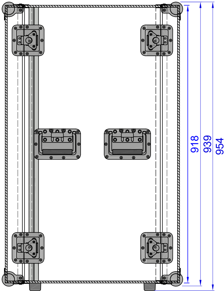
Seitenansicht / sideview
