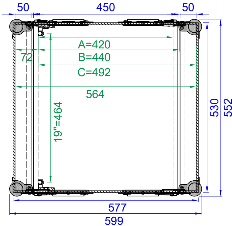
Draufsicht / topview
