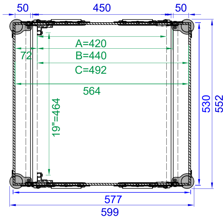
Draufsicht / topview
