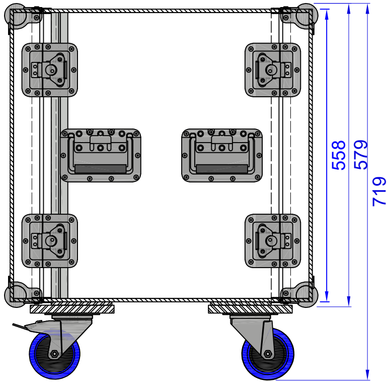
Seitenansicht / sideview
