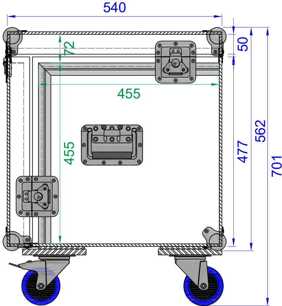
Seitenansicht / sideview
