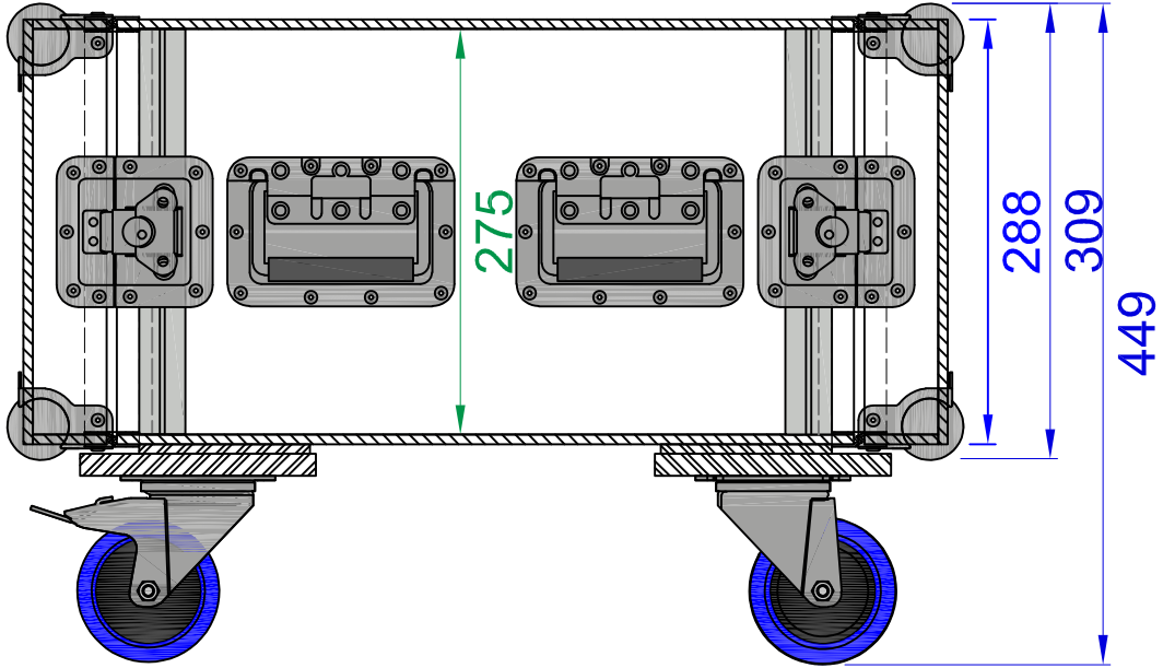
Seitenansicht / sideview
