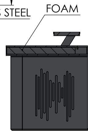
SECTION AS-AS SCALE 1 : 20
