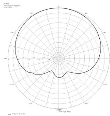
Polardiagramm @ 1 kHz
