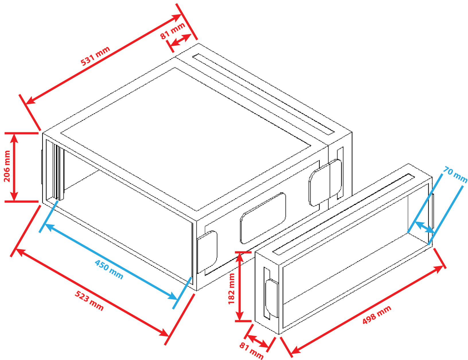
Case 4U Double Door Profi
