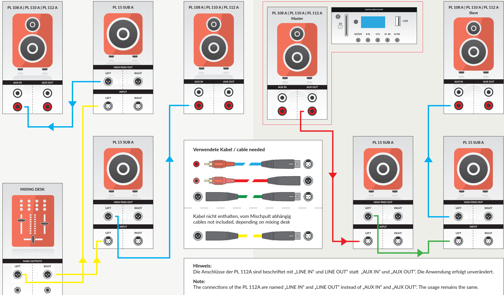
Variante 1: Stereo mit externem Mischpult / variation 1: stereo with external mixing desk
